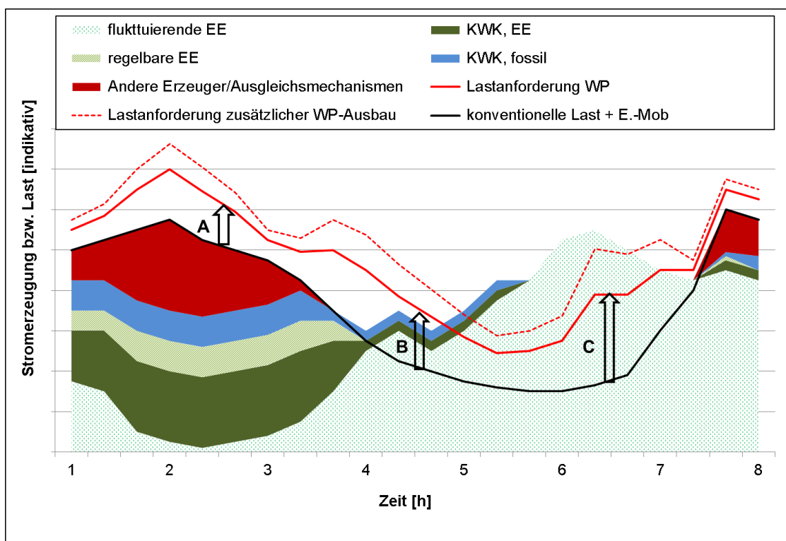
Abbildung 9: Indikative Darstellung des Strommixes für Wärmepumpenstrom für typische Situationen
