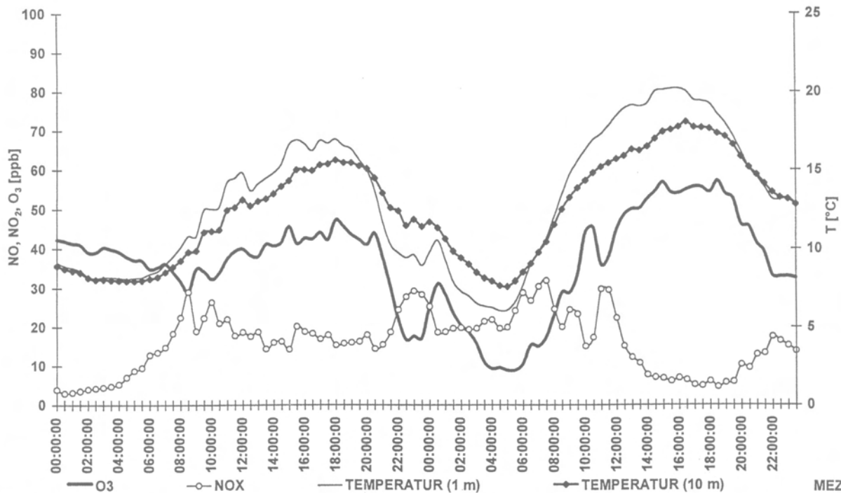
Abb. 1: Tagesgang der O 3 - und NO x -Konzentrationen, der Lufttemperatur (1 und 10 m Höhe ü. Gr.) am 28./29.05.1997 im Grugapark der Stadt Essen (30-min-Mittelwerte, Datenbasis: 10-s-Werte)
