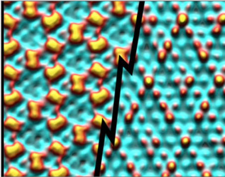
Die beiden Phasen von Kohlenstoffmonoxid (CO) auf Kupfer (Cu) im Nanometermaßstab, aufgenommen mit einem Rastertunnelmikroskop. © CENIDE/AG Möller
