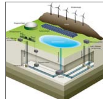
Pumpspeicherkraftwerk. © UDE
